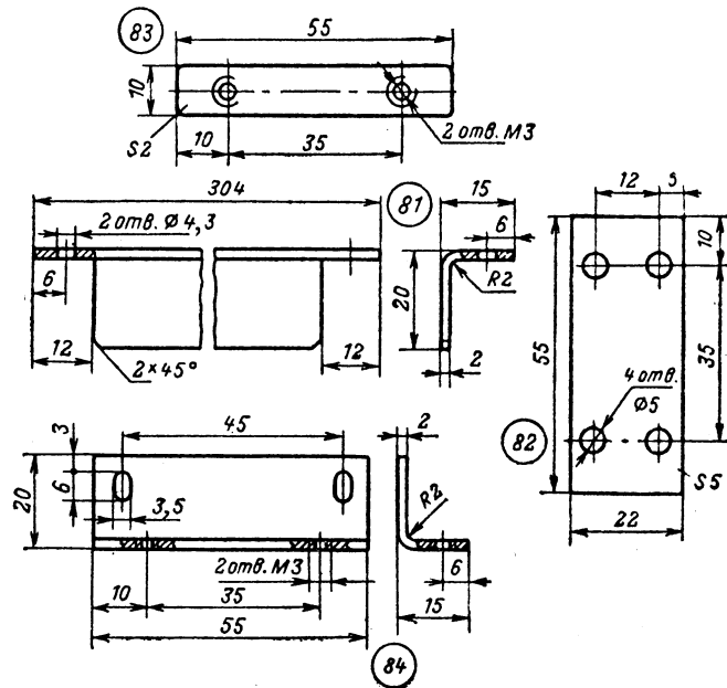
Рис. 13. Детали проигрывателя.
